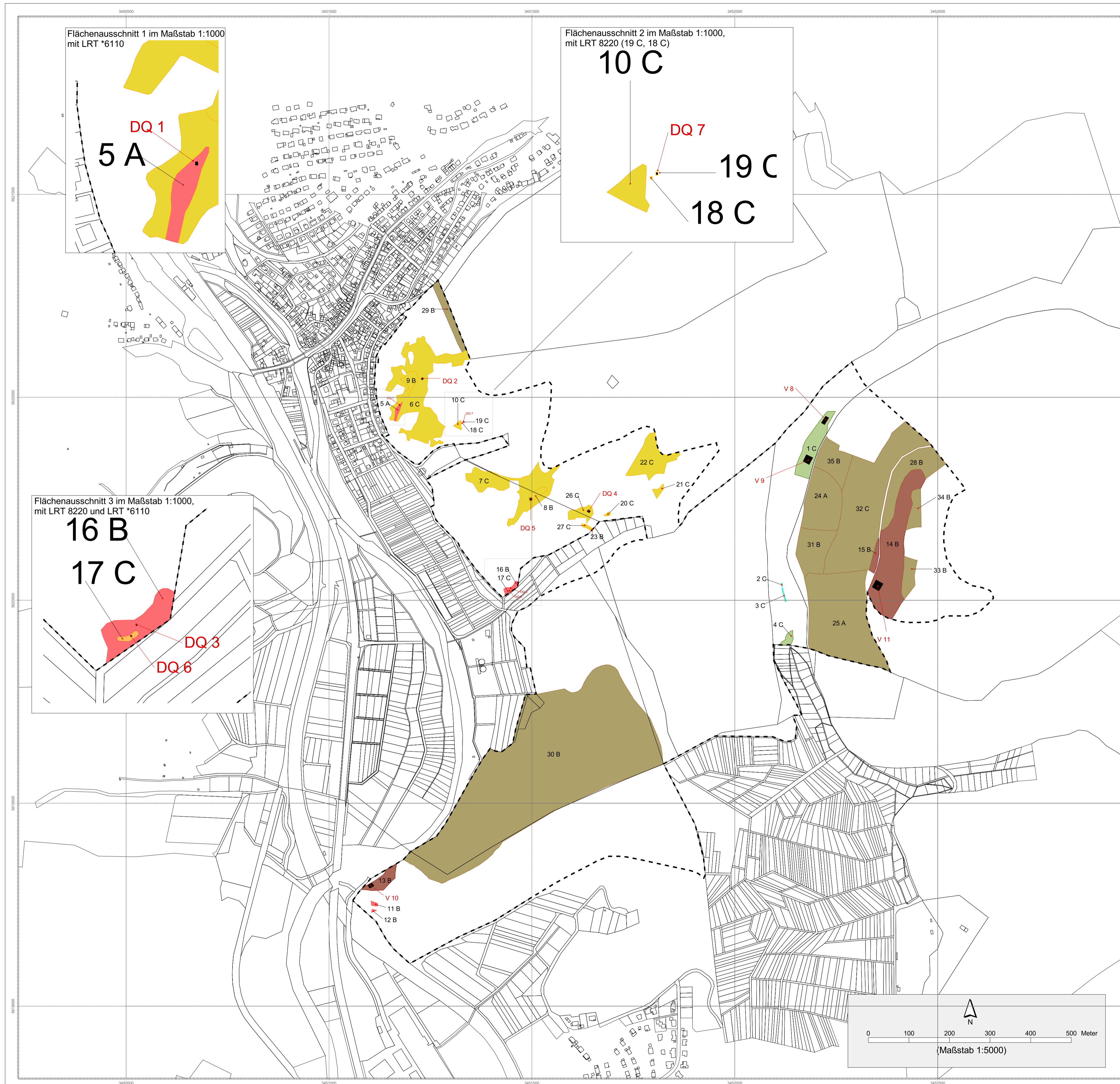
Karte 1: FFH-Lebensraumtypen in Wertstufen inkl. Lage der Dauerbeobachtungsflächen
